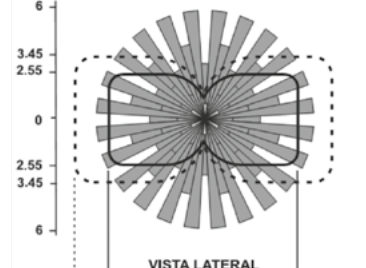
OSC10-MOW/ODC10-MOW Campo de visión en metros
