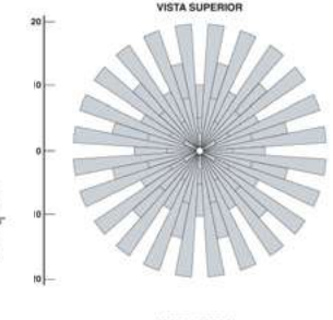
OSWWV-IOW Campo de visión en metros
