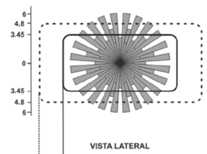
OSC20-MOW/ODC20-MOW Campo de visión en metros
