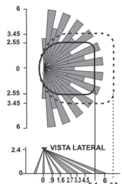
OSC05-MOW/ODC05-MOW Campo de visión en metros
