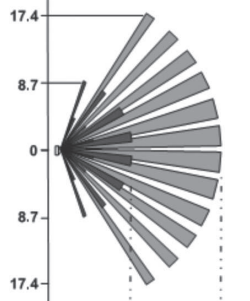
VISTA LATERAL OSWWV-IOW Campo de visión en metros
