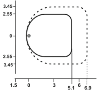
OSC05-UOW/ODC05-UOW Campo de visión en metros
