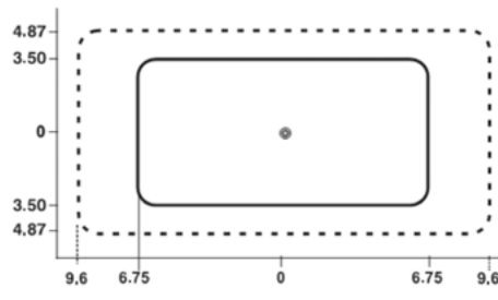
OSC20-UOW/ODC20-VOW Campo de visión en metros
