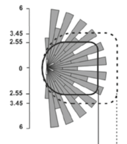
OSC05-MOW/ODC05-M0W Campo de visión en metros
