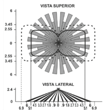
OSC10-M0W/ODC10-M0W Campo de visión en metros
