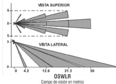
OSWLR Campo de visión en metros
