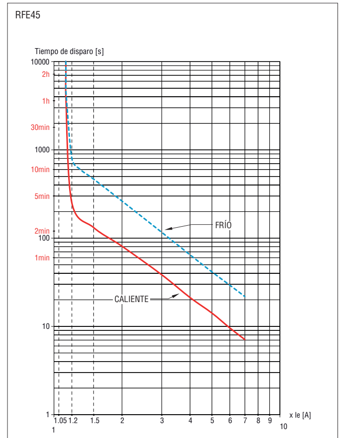
Funcionamiento equilibrado en 3 fases; clase 30
