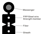
Fibra óptica DROP exterior
