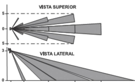
OSWLR Campo de visión en metros
