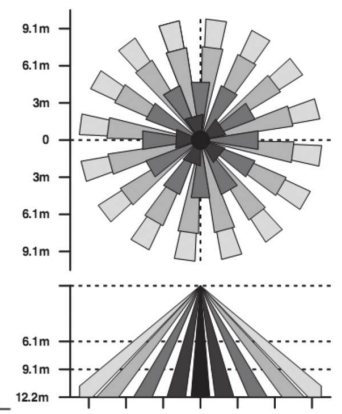
OSFHU-ITW/OSFHU-CTW Campo de visión en metros
