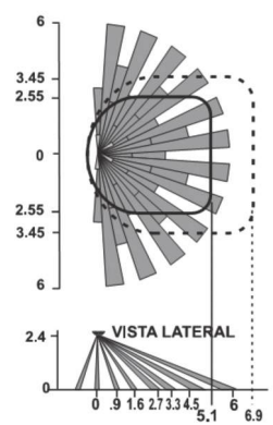
OSC05-MOW/ODC05-MOW Campo de visión en metros
