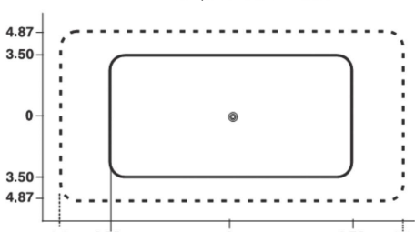
OSC20-UOW/ODC20-VOW Campo de visión en metros
