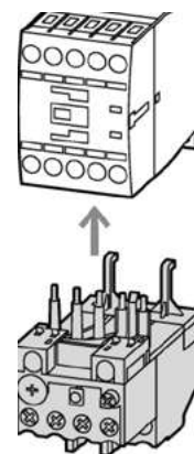
MONTAJE DIRECTO DILM7...15 + ZB12...
